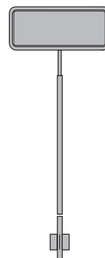
Rørrammestander Højde fra jord til underkant af skilt: 220 cm.
